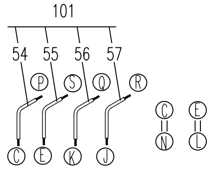
Wiring scheme
